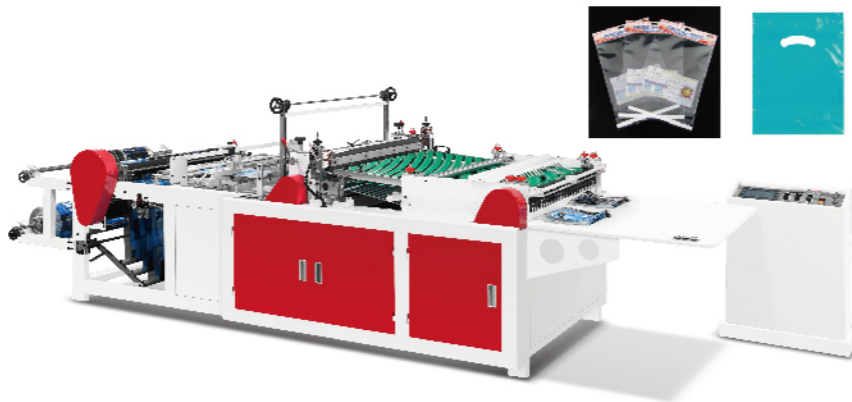
Hole puncher 打孔机 Servo Motor
