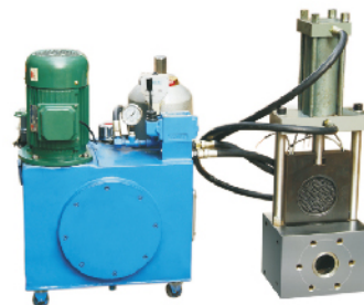
Hydraulic Filter Changer 液压换网器
